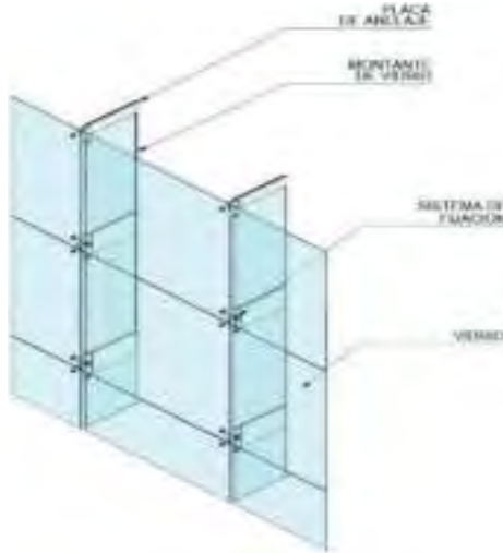
Figura 4. Sistema suspendido
