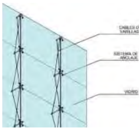
Figura 1. Sistema pretensado
